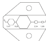
Crimpeinsatz profil
