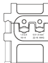
Crimpeinsatz profil
