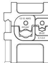
Crimpeinsatz profil
