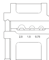
Crimpeinsatz profil
