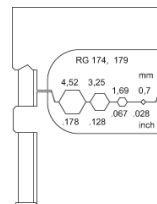
Crimpeinsatz profil
