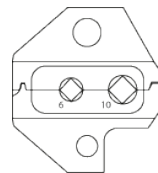
Perfil de matriz
