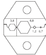
ダイの断面
