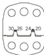
ダイの断面
