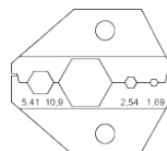
ダイの断面
