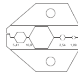
Die profile
